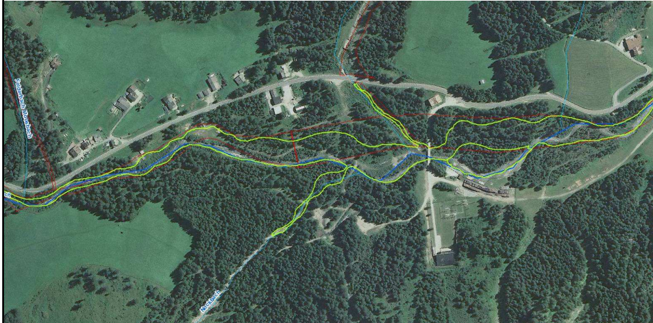
Revitalisierung Mühlwalderbach – Rivitalizzazione Rio Molini
