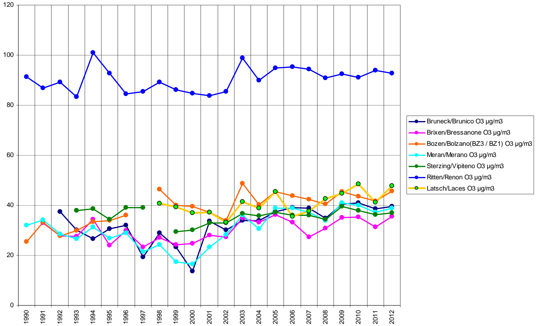
O3 - Jahresmittelwerte/medie annuali [ \mu\text{g}/\text{m}^3 ]
