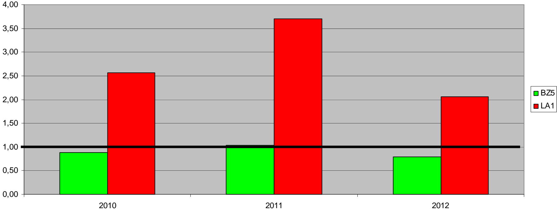
PAK Jahresmittelwert- IPA media annuale (ng/m3)
