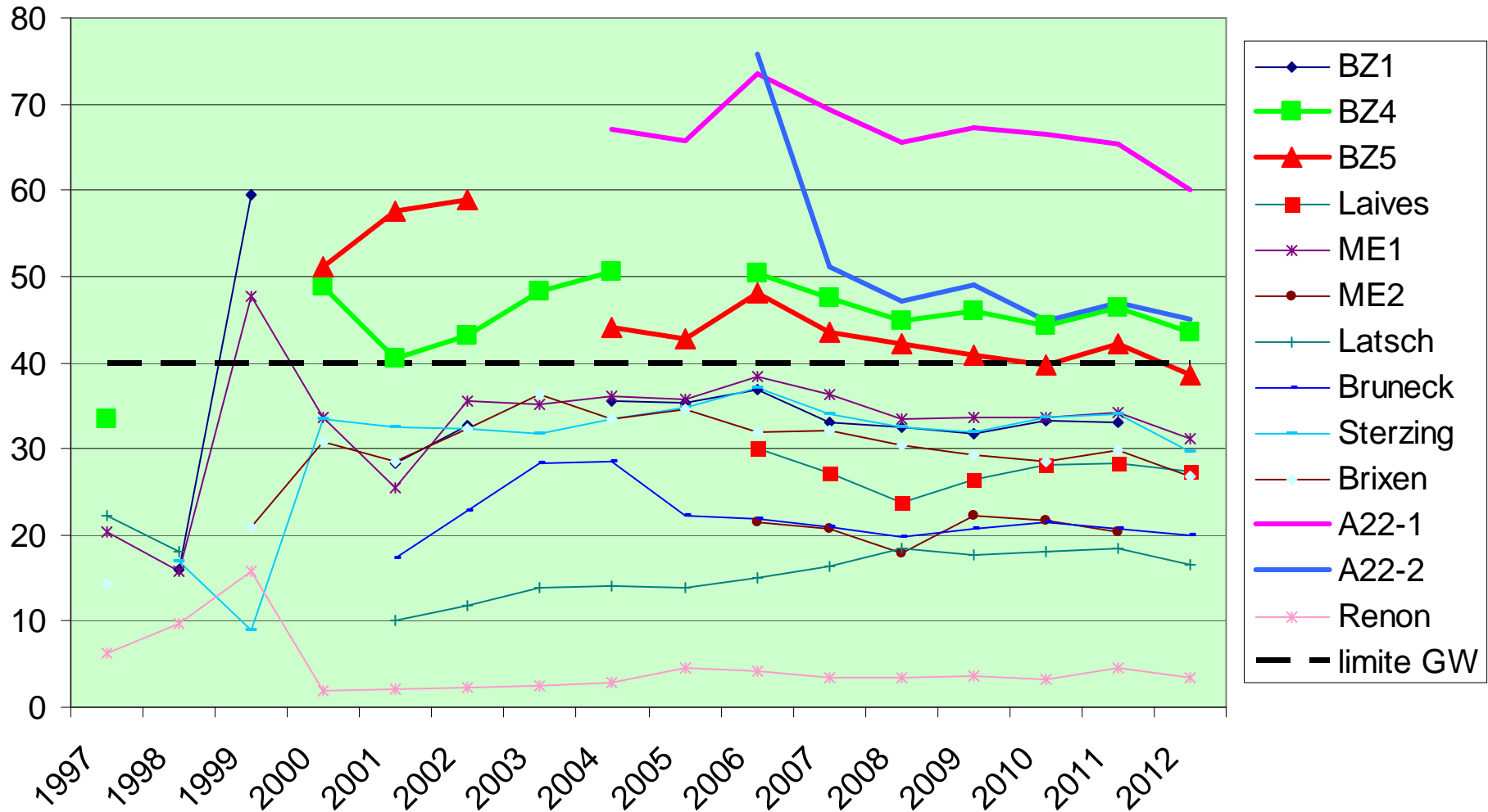
NO2 - Jahresmittelwerte/medie annuali [ \mu\text{g}/\text{m}^3 ]
