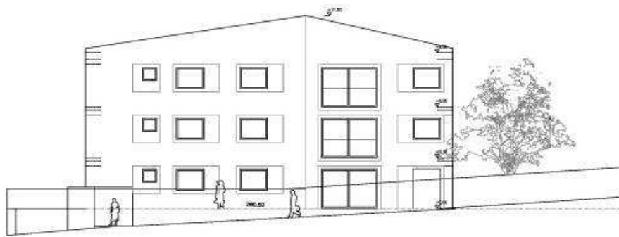
Westansicht
