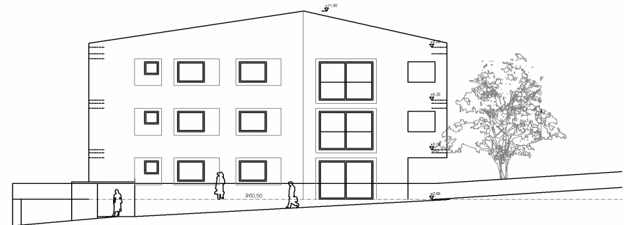
Westansicht
